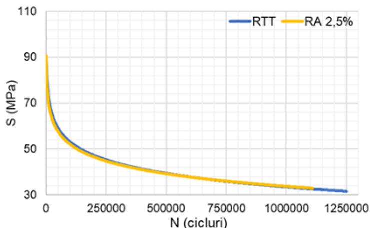
Figura 3.5. Curbele lui Wöhler pentru RTT și RA 2,5%.
