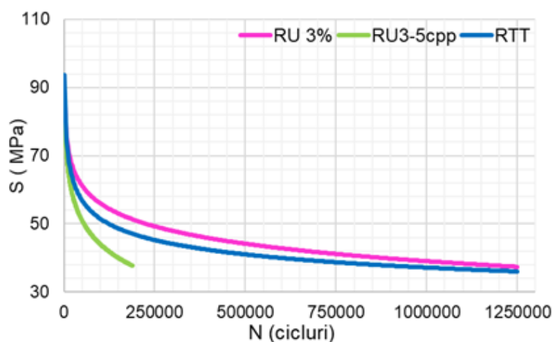
Figura 3. 12. Compararea curbelor S-N pentru epruvetele RU 3% și RU3-5cpp.
