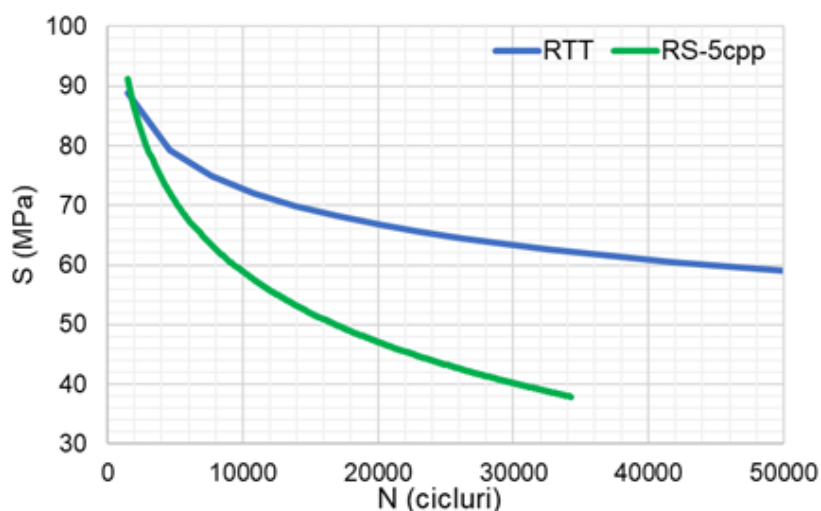
Figura 3. 10. Comparație între curbele S-N ale epruvetelor RTT și RS-5cpp.
