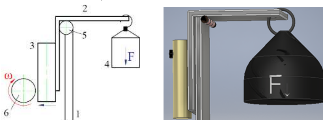
Figura 2. 5. Dispozitiv pentru realizarea uzurii prin frecare cu alunecare.
