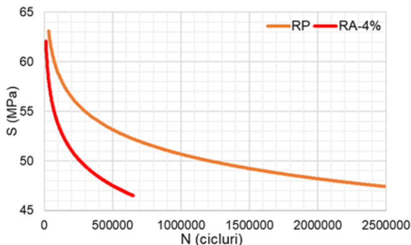
Figura 3. 4. Curbele lui Wöhler pentru RP și RA 4 %.
