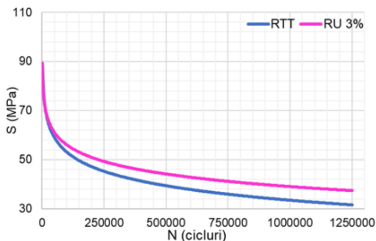
Figura 3. 7. Curbele lui Wöhler pentru RTT și RU 3%.
