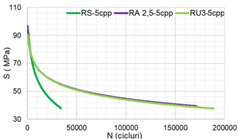
Figura 3. 13. Comparație între curbele S-N ale epruvetelor RS-5cpp, RA2,5-5cpp și RU3-5cpp.
