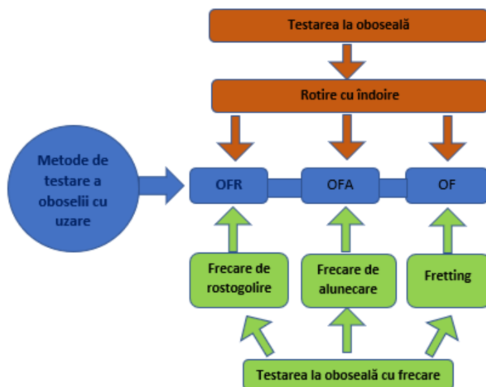
Figura 2. 4. Dezvoltarea metodelor de testare a obosealii cu uzare în timpul mișcării principale de rotație: OFR - oboseală cu frecare de rulare; OFA - oboseală cu frecare de alunecare; OF - oboseala la fretting [55],[70]
