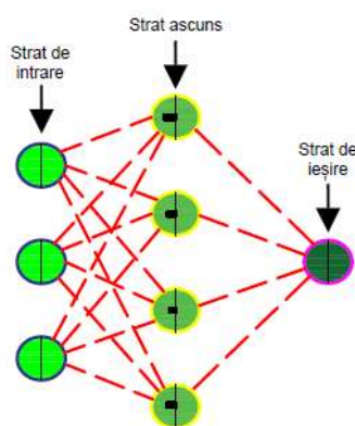
Figura 4. 1 Rețea neuronală cu structură „Feed-forward”
