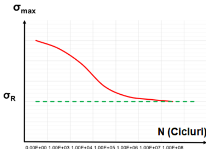
Figura 1. 1. Curba lui Wöbler specifică unor oțeluri. [38]
