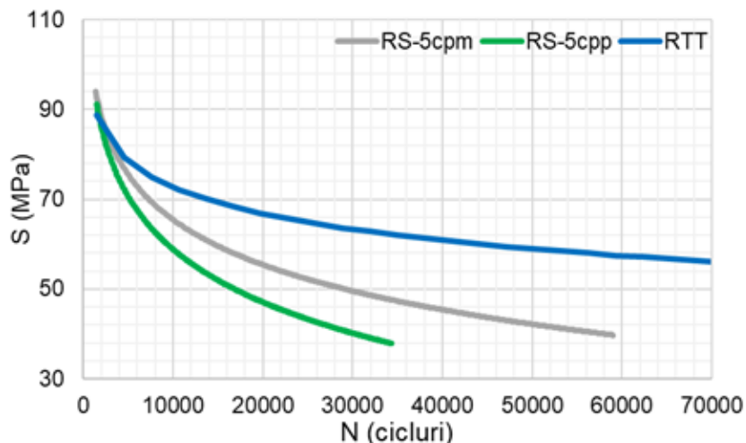
Figura 3. 14. Comparație între epruvetele RTT, RS-5cpm și RS5-Mp.
