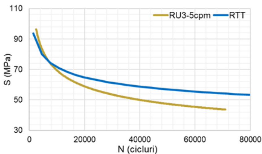
Figura 3. 17. Curba S-N pentru epruvetele RU3-5cpm.
