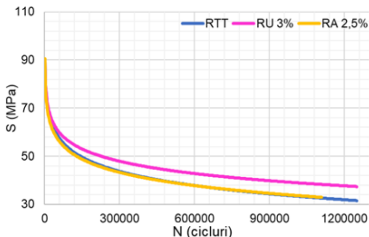
Figura 3. 8. Comparație între epruvetele RTT, RU 3% și RA 2,5%.
