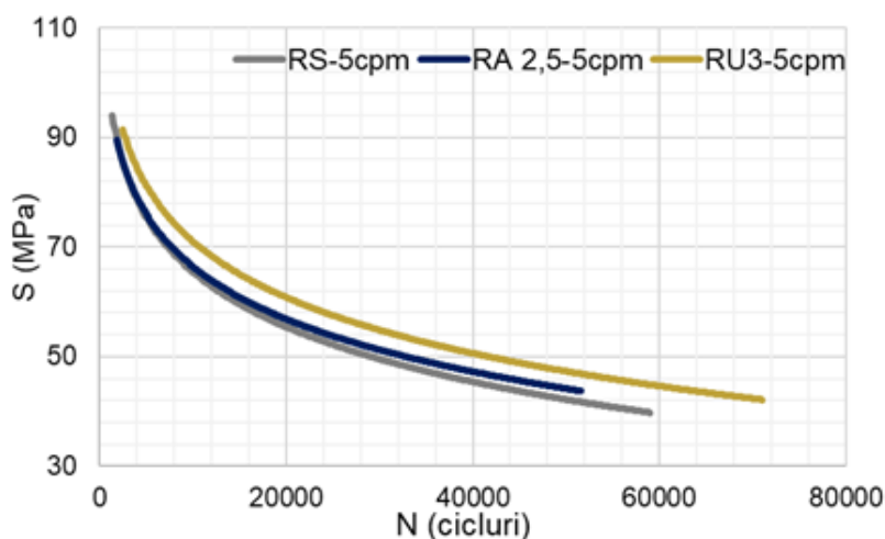
Figura 3. 19. Comparație între RS-5cpm, RA2,5%-cpm și RU3-5cpm.
